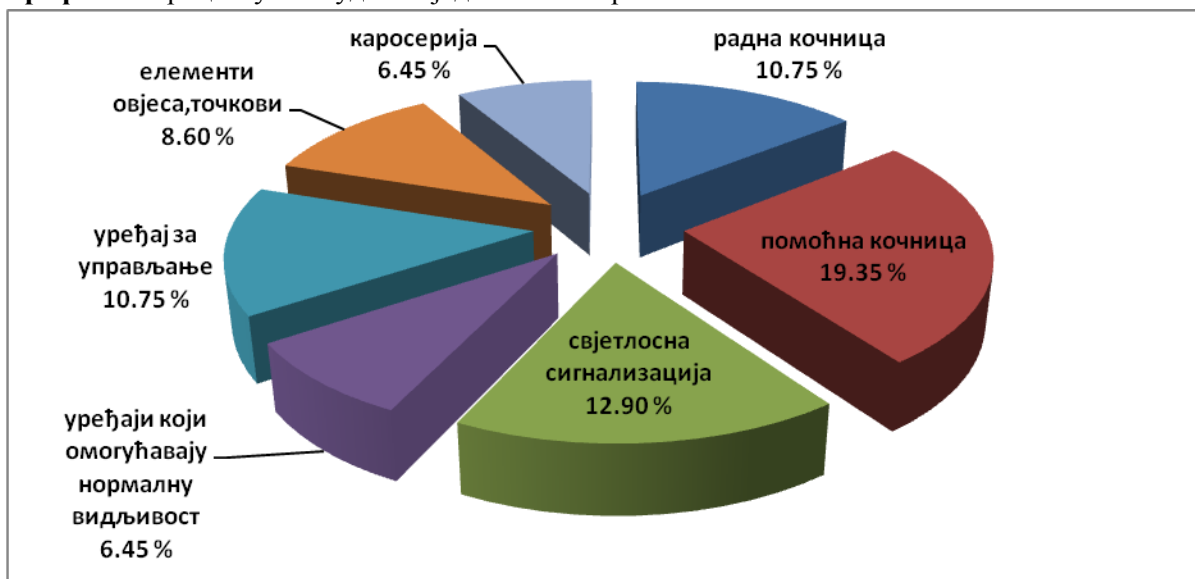
График 4. Процентуални удио појединих неисправности на испитаним возилима
